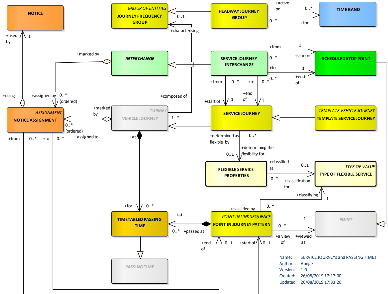
Figure 2 – Vehicle Journey, Passing Times et Interchanges – Modèle conceptuel
