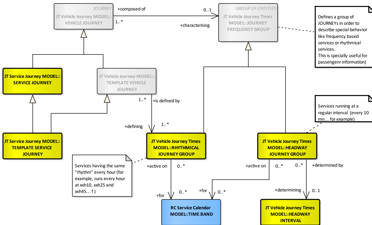
Figure 4 – Template Service Journey – Modèle conceptuel
